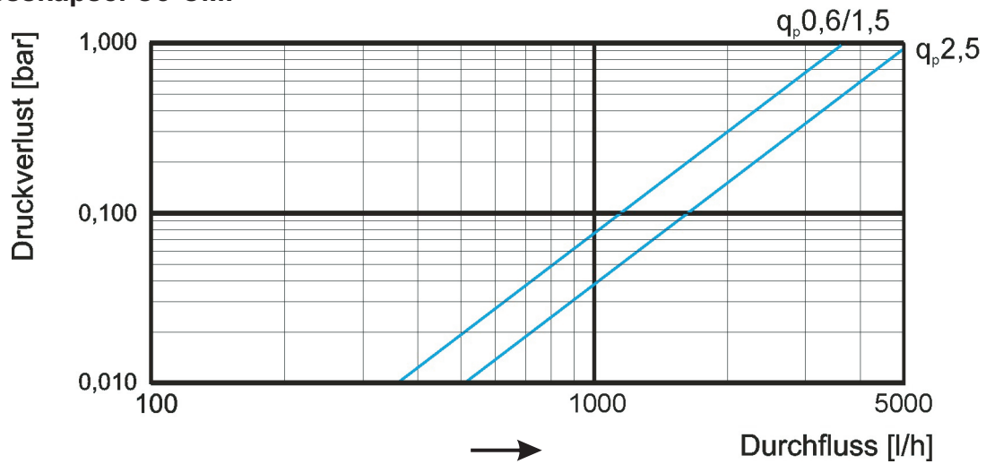
Einstrahl-Durchflusssensor C5-ISF
