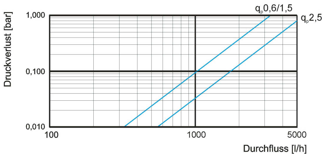
Einstrahl-Durchflusssensor C5-ISF
